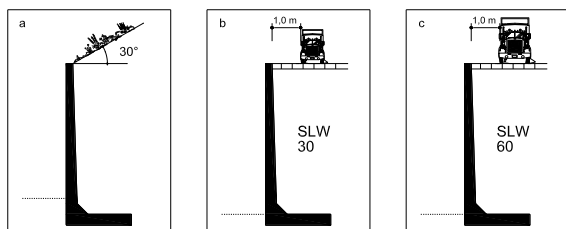
Lastfall 2
