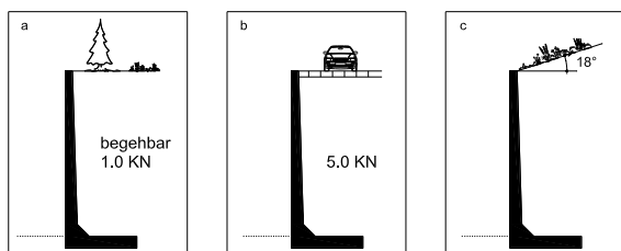
Lastfall 1
