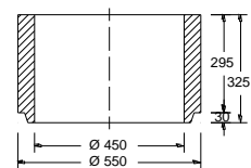
Muffen Teil 3a /3l*/3kg**
