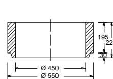
Boden Teil 1g /1gL*/1kgk**
