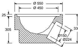
Boden Teil 1a /1l*/1kg**
