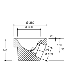
Boden T.21 u. T.21 m.KG
