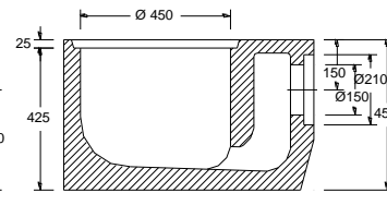
Boden Teil 1g /1gL*/1kgk**
