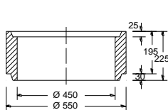
Boden Teil 1a /1l*/1kg**
