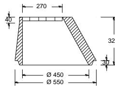
Schaft Teil 5c
