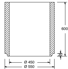
Schaft Teil 5d
