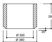
Schaft kurz T.26
