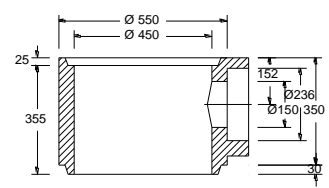
Muffen Teil 3a /3l*/3kg**
