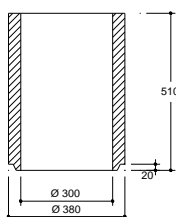
Schaft lang T.25
