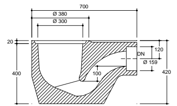
Boden mit Geruchsverschluss T.23 u. T.23 m.KG
